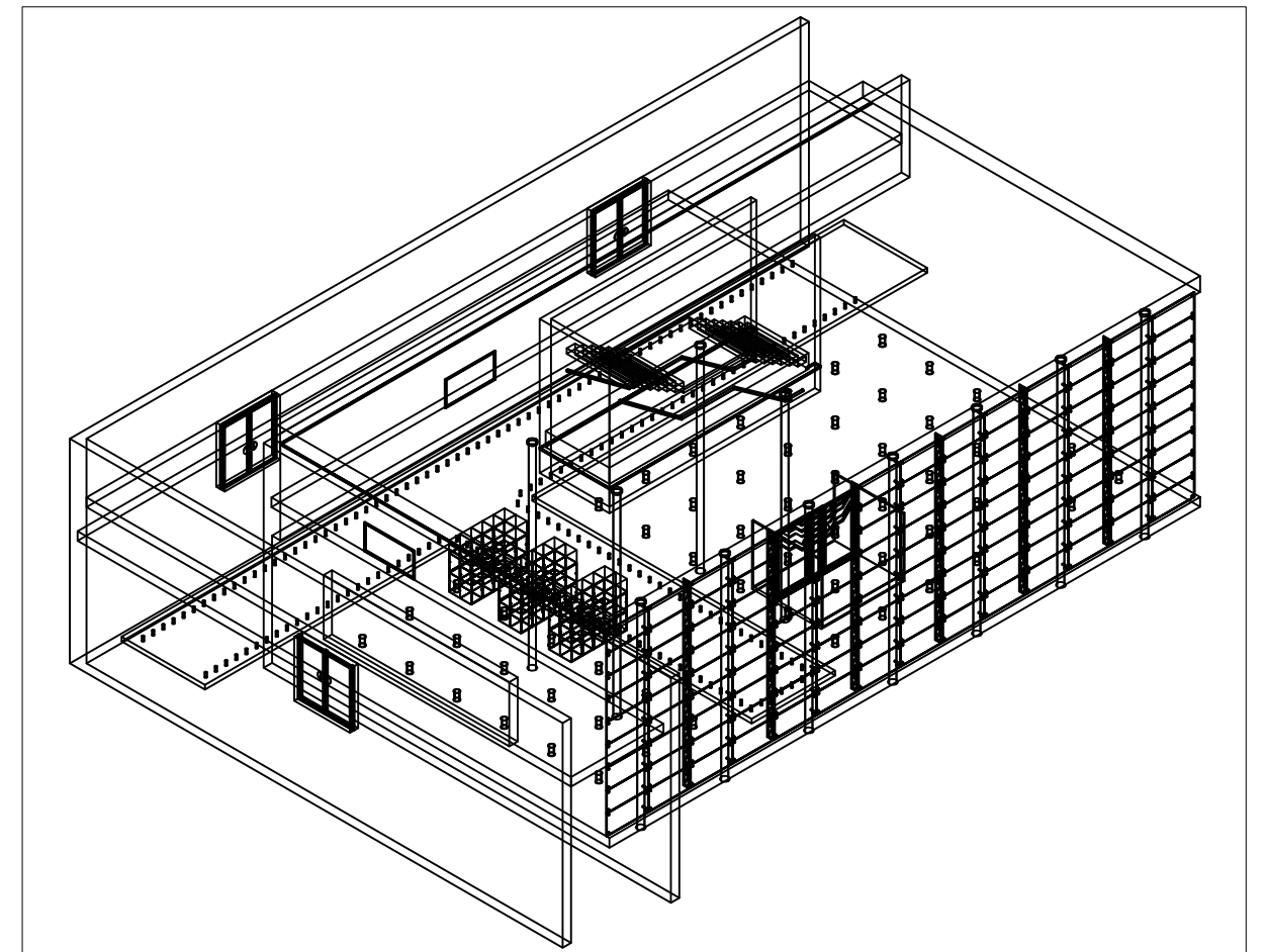
Isometrische Ansicht aus AutoCAD
